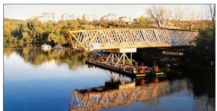
Der Bau der Fußgängerbrücke über den Neckar im Jahr 1988.
